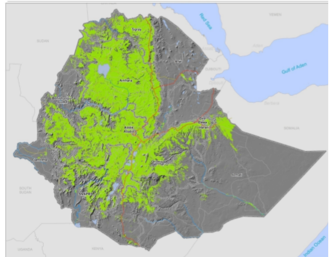
NUDSP - Cropland 2014
